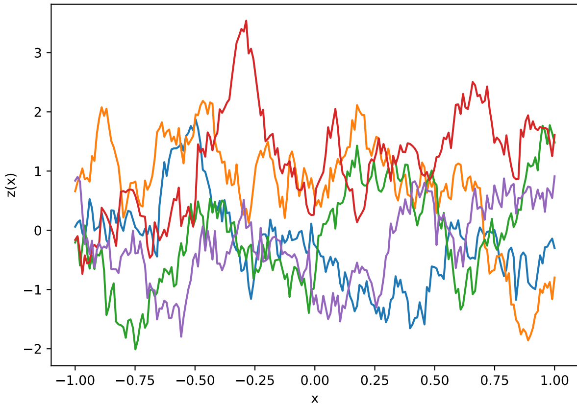
GP - Ornstein-Uhlenbeck kernel
